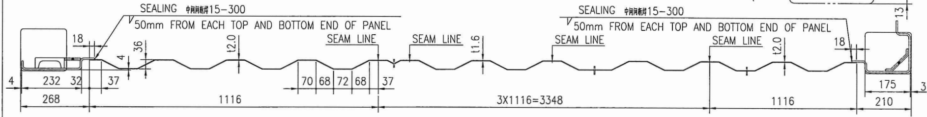
SECTION A-A 1:10
