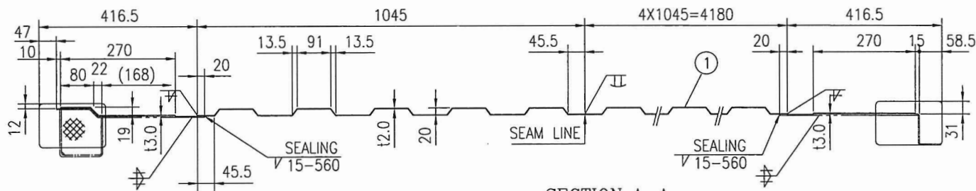
SECTION A-A 1:10
